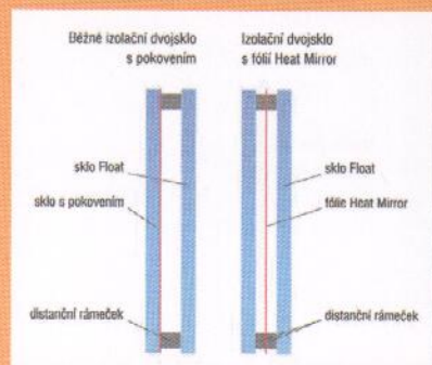
Obr. 6 Schéma umístění fólie Heat Mirror
