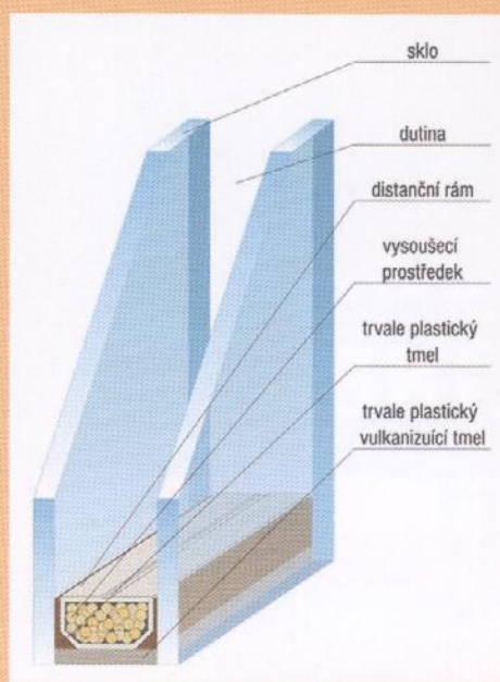
Obr. 3 Teplé rámečky by měly být u oken pro pasivní domy samozřejmostí. Na obrázku je řez zasklením s teplým distančním rámečkem
